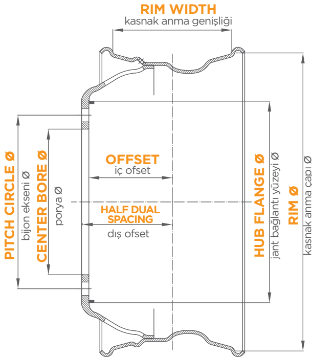
Alive Disc Wheel for dual fitment with 15° drop centre rim for tubeless tyres Çift bağlantıya uygun 15° topuk açılı dıştan sübaplı tubeless jant
