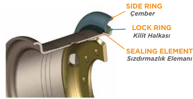
FLAT BASE TUBELESS WHEEL WITH SEALING ELEMENT Alçak Düz Tabanlı Tubeless Jant (Sızdırmazlık Elemanlı)
